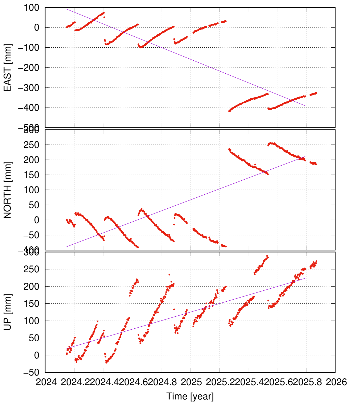
ORFC ( , ) time series (IGb20) ve = +- ; vn = +- ; vu = +- mm/yr
